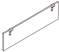
MFC Modesty Panel Fixed on Top 三聚氰胺板前挡板·台底固定 W: 900, 1140, 1240, 1340 T: 16 H: 350
