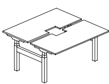
Bench 双边共享升降台 (3节脚) W: 1400,1500,1600,1800 D: 1200,1400,1600 H: 625-1275
