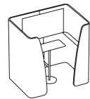
Standing Suite 站立式休闲间 W1800 D1300 H1800
