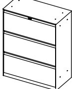
Base 下置 W900 D450 H784/1136
