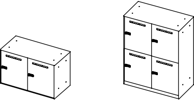
Upper 上置 W900 D450 H556.5 Base 下置 W900 D450 H1136
