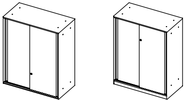
Upper 上置 W900 D450 H724/1076 Base 下置 W900 D450 H784/1136
